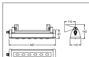
Wandanbau mit Wandhalterung, schwenkbar
