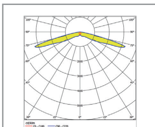
Lichtverteilungskurve
